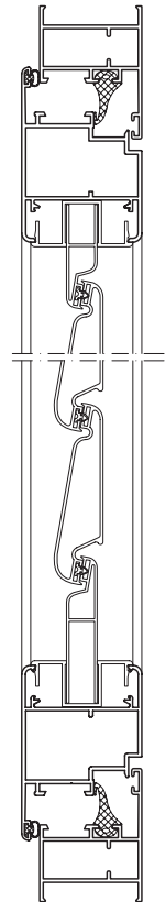
Sección característica
